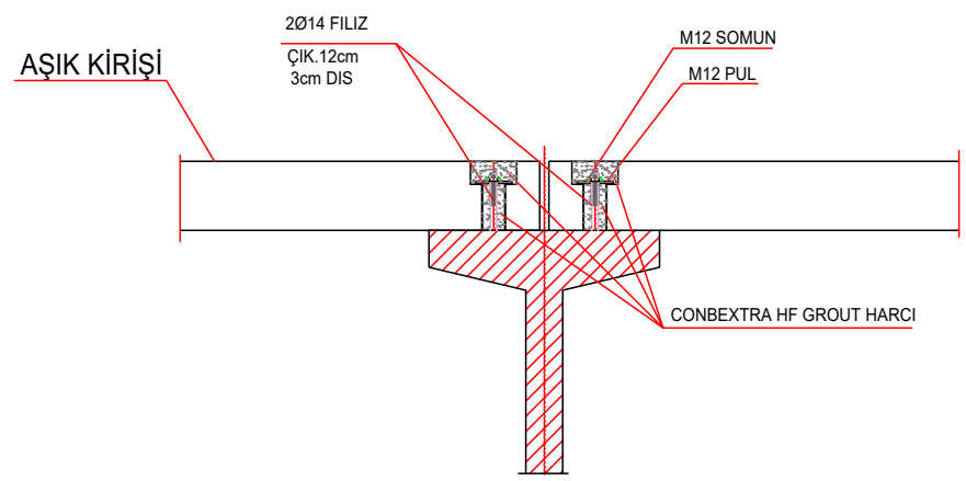
AŞIK-MAKAS BAĞLANTI DETAYI
