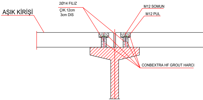
AŞIK-MAKAS BAĞLANTI DETAYI
