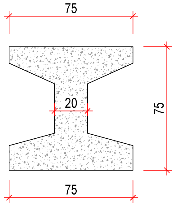
a-a kesiti
