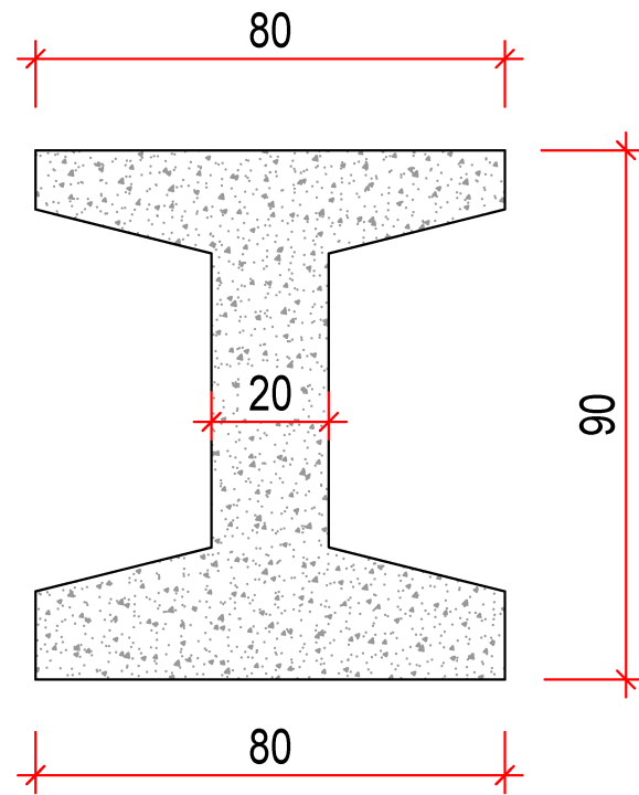
a-a kesiti
