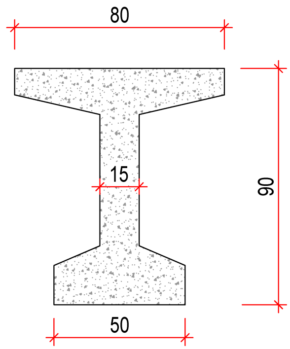
a-a kesiti
