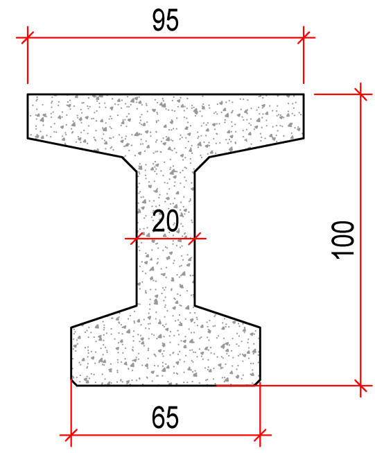
a-a kesiti
