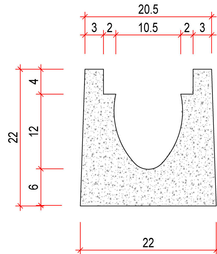
b-b kesiti
