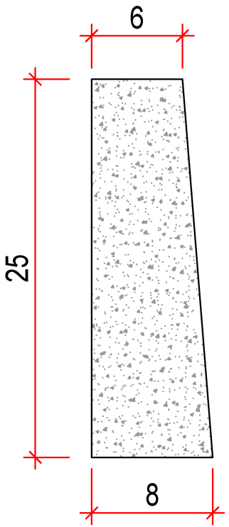
b-b kesiti
