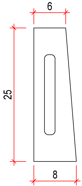
a-a görünüşü
