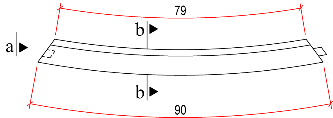
ÜST GÖRÜNÜŞ
